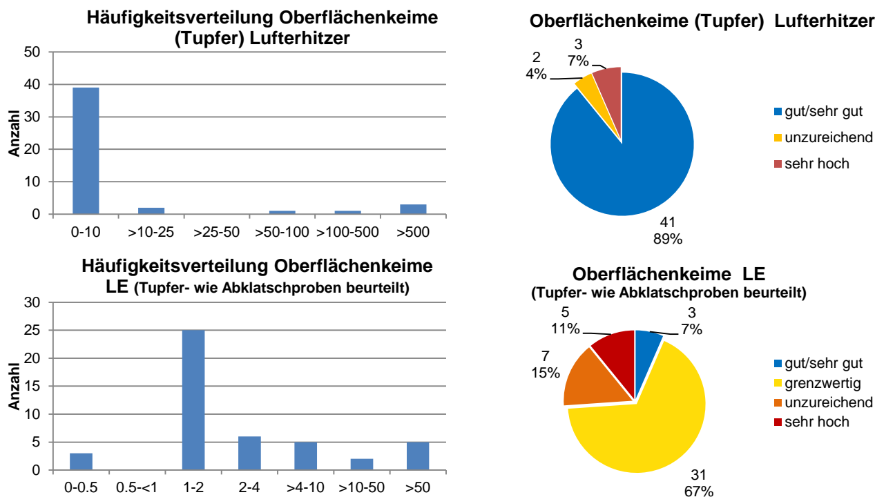
Abb. 89: Beurteilung aller Tupferproben am Luftheritzer (n=46). Oben: Beurteilung nach internem Standard diesen Projekts (siehe ); Unten: Anwendung der Beurteilungswerte für Abklatsche der SWKI-Richtlinie VA104-02.
