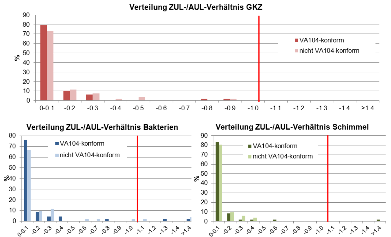
Abb. 53: Häufigkeitsverteilung des Verhältnisses Zuluft-/Aussenluftkonzentration bezüglich Gesamtkeimzahl (GKZ), Schimmelpilzsporen und Bakterien bei mit SWKI VA104-01 konformen und nicht konformen Filterstufen mit Anforderung SWKI-Richtlinie VA104-01 (rote Linie)
