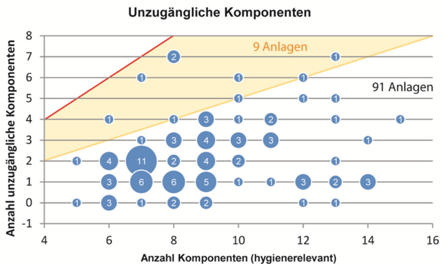
Abb. 22: Anzahl unzugängliche Komponenten zur Gesamtzahl der hygienerlevanten Komponenten der entsprechenden RLT-Anlage. Die Blasenfläche entspricht der Anzahl Anlagen mit gleicher Paarung. Orange hinterlegt: Anlagen, deren Anteil unzugänglicher Bauteile 50 % und mehr beträgt.
