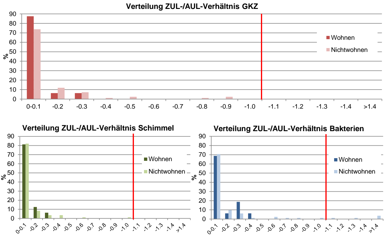
Abb. 42: Häufigkeitsverteilung des Verhältnisses Zuluft-/ Aussenluftkonzentration bezüglich Gesamtkeimzahl (GKZ), Schimmelpilzsporen und Bakterien bei Wohngebäuden (n=14) und Nichtwohngebäuden (n=86) mit Anforderung SWKI-Richtlinie VA104-01 (rote Linie)
