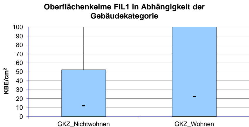
Abb. 39: Statistische Auswertung der Oberflächenkeime (GKZ) in Abhängigkeit vom Gebäudetyp (Wohnbauten/Nichtwohnbauten). Die Box entspricht dem 10. bzw. 90. Perzentil, die Strichenden dem Minimal- bzw. Maximalwert und der Querstrich dem arithmetischen Mittelwert.
