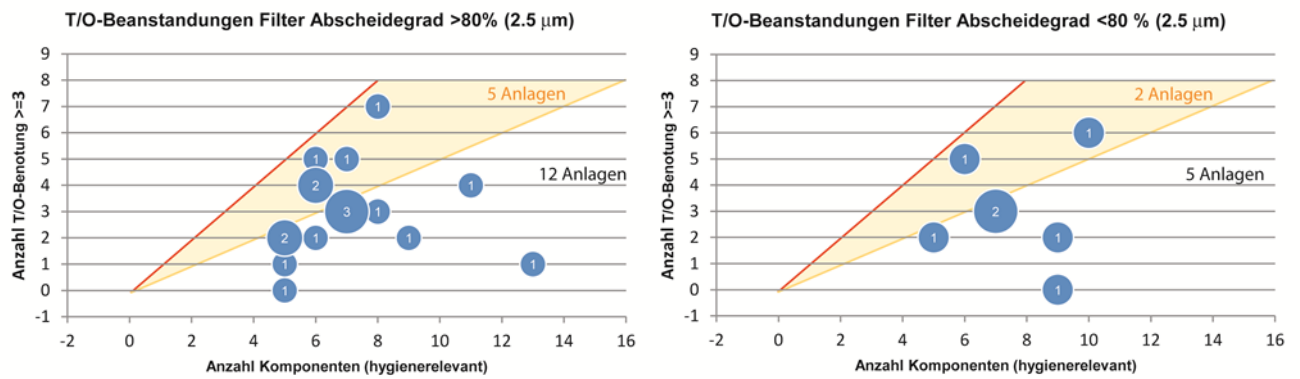
Abb. 55: Anzahl technisch-optische Beanstandungen (ohne unzugängliche Komponenten) in Abhängigkeit zur Gesamtzahl der hygienerlevanten Komponenten der entsprechenden RLT-Anlage und zum Abscheidegrad.
