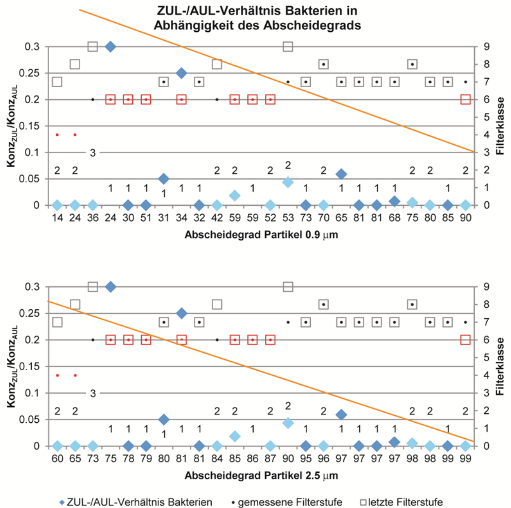
Abb. 58: Zuluft-/Aussenluftverhältnis der Bakterienkonzentration in Abhängigkeit vom Abscheidegrad
