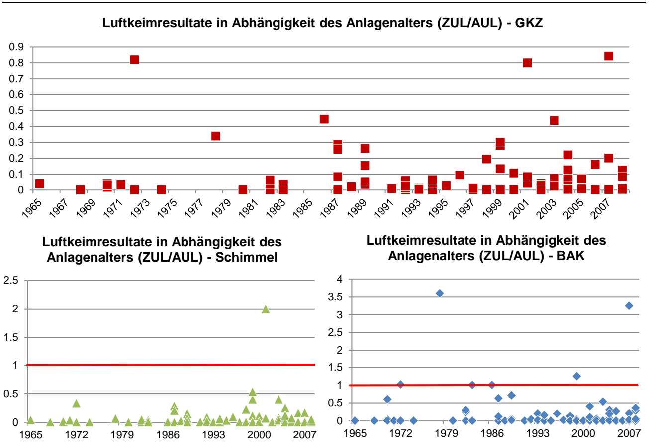
Abb. 69: Verhältnis Zuluft-/Aussenluftkonzentration bezüglich Gesamtkeimzahl (GKZ), Schimmelpilzsporen und Bakterien in Abhängigkeit vom Anlagenalter mit Anforderung SWKI-Richtlinie VA104-01 (rote Linie)
