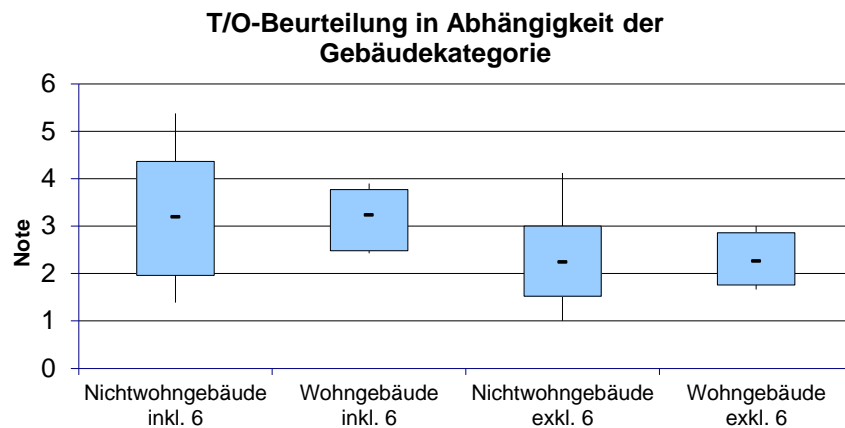
Abb. 36: Statistische Auswertung der T/O-Gesamtnote hygienerrelevanter Komponenten in Abhängigkeit vom Gebäudetyp (Wohnbauten/Nichtwohnbauten). Die Box entspricht dem 10. bzw. 90. Perzentil, die Strichenden dem Minimal- bzw. Maximalwert und der Querstrich dem arithmetischen Mittelwert.
