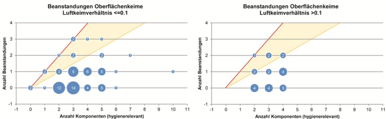
Abb. 61: Anzahl Beanstandungen bezüglich Oberflächenkeimen (Abklatsche und Tupferproben) in Abhängigkeit zur Gesamtzahl der Messorte der entsprechenden RLT-Anlage und des Luftkeimverhältnisses.
