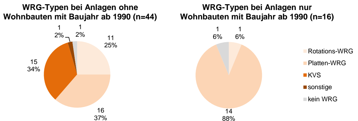
Abb. 84: Verteilung der WRG-Typen in Abhängigkeit vom Baujahr der Anlage und vom Gebäudetyp (Nichtwohngebäude/Wohngebäude)
