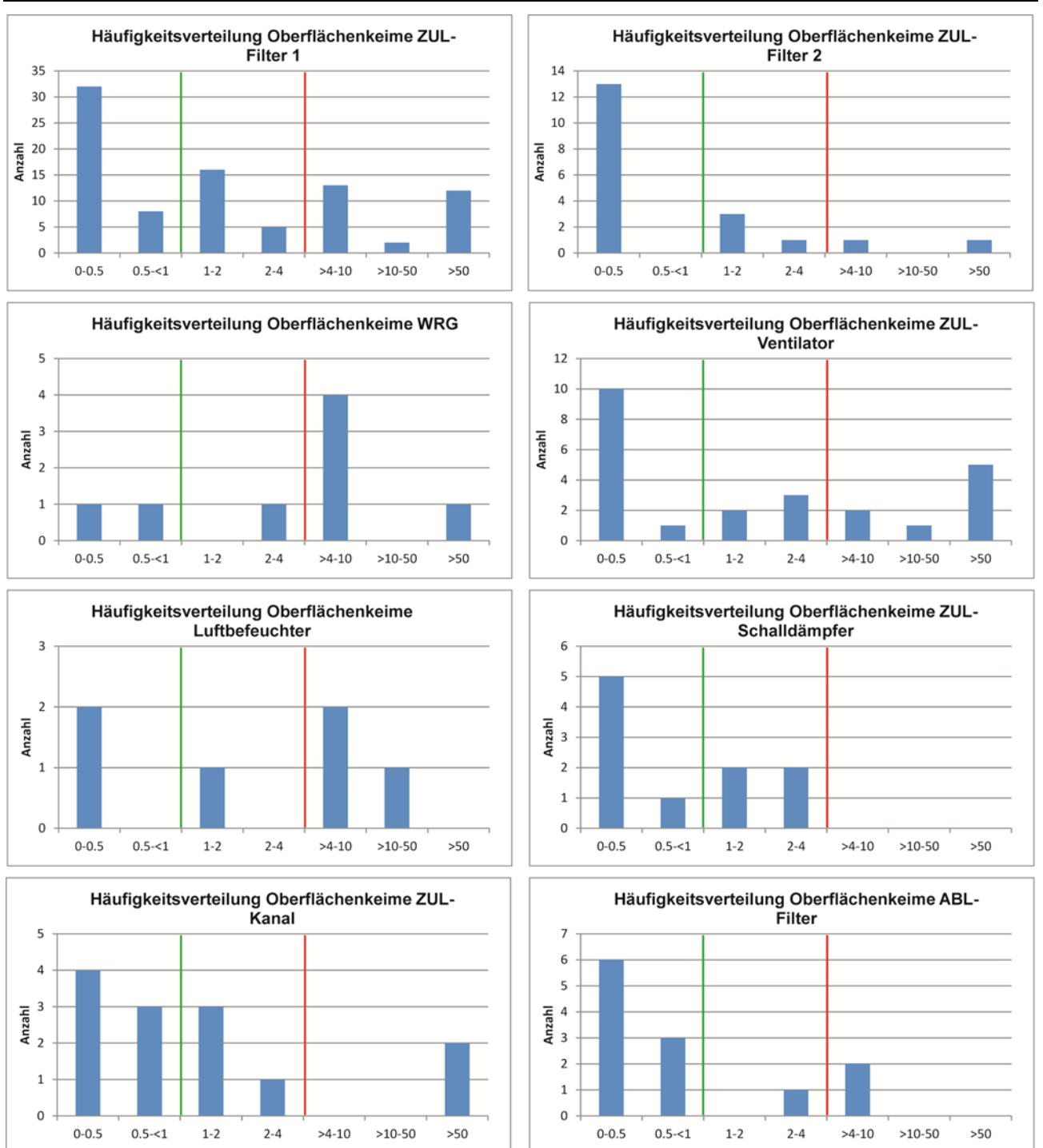
Abb. 23: Häufigkeitsverteilung der nachgewiesenen Oberflächenkeime (GKZ in KBE/cm 2 ) von Abklatschproben in den jeweiligen Bauteilen. Rote Linie: Erfahrungswerte zur Beurteilung gemäss SWKI VA104-02 (rechts → unzureichend), grüne Linie: Erfahrungswerte (links → gut bis sehr gut)
