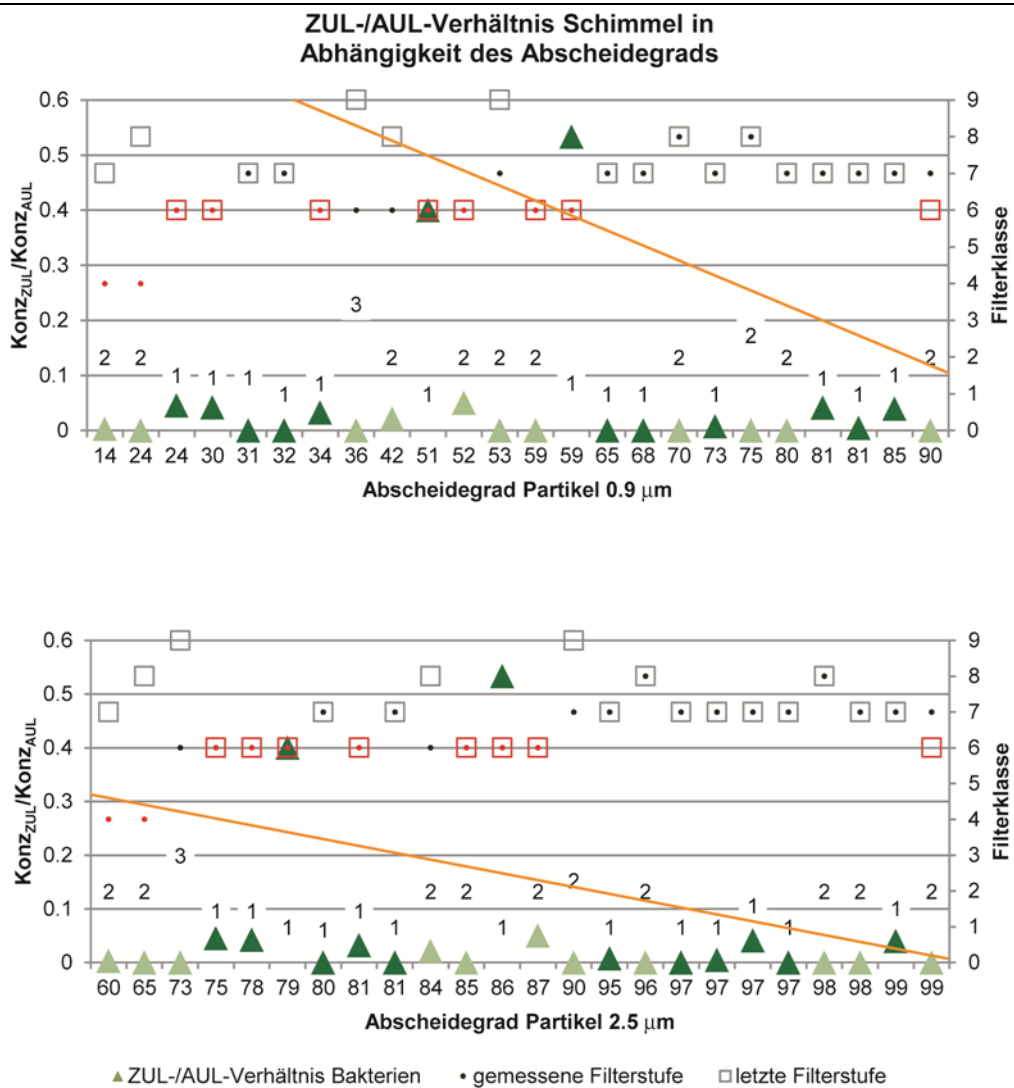
Abb. 57: Zuluft-/Aussenluftverhältnis der Schimmelpilzkonzentration in Abhängigkeit vom Abscheidegrad
