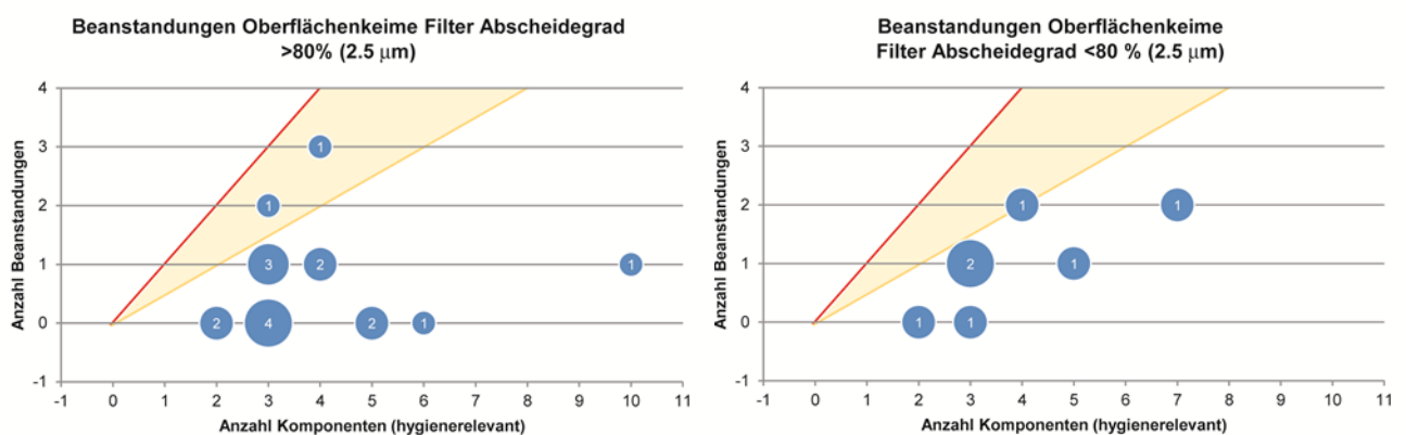
Abb. 56: Anzahl Beanstandungen bezüglich Oberflächenkeimen (Abklatsche und Tupferproben) in Abhängigkeit zur Gesamtzahl der Messorte der entsprechenden RLT-Anlage und zum Abscheidegrad.
