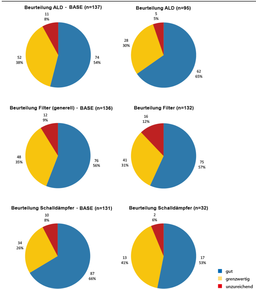
Abb. 32: Vergleich der T/O-Bewertungen von Aussenluftdurchlass (ALD); Zuluffiltern (FIL) und Schalldämpfern der BASE-Studie (linke Kreisdiagramme) mit der vorliegenden Untersuchung (rechte Kreisdiagramme).
