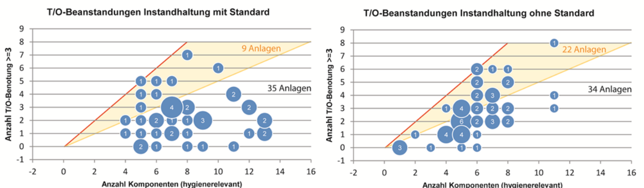
Abb. 74: Anzahl technisch-optische Beanstandungen (ohne unzugängliche Komponenten) in Abhängigkeit zur Gesamtzahl der hygienerelevanten Komponenten der entsprechenden RLT-Anlage und der Anwendung eines anerkannten Standards bei der Instandhaltung.
