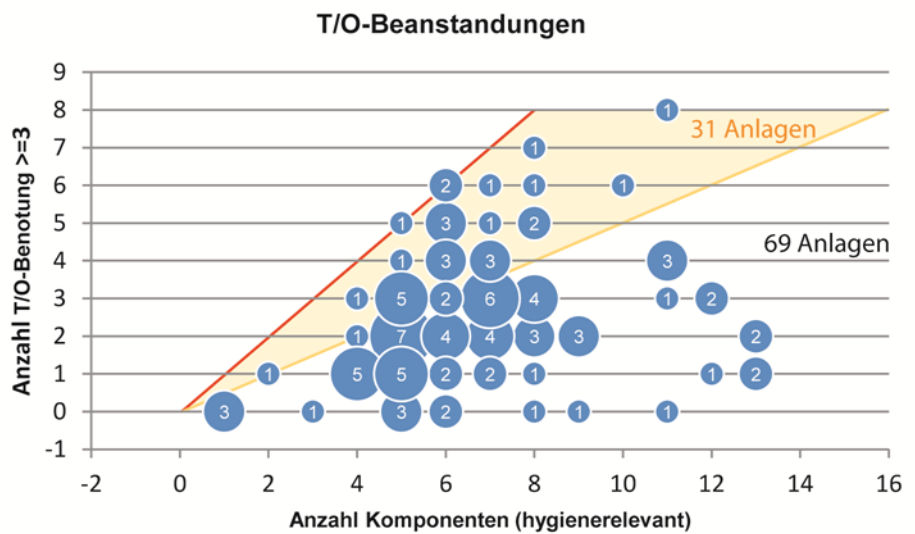
Abb. 21: Anzahl technisch-optische Beanstandungen (ohne unzugängliche Komponenten) zur Gesamtzahl der hygienerlevanten Komponenten der entsprechenden RLT-Anlage. Die Blasenfläche entspricht der Anzahl Anlagen mit gleicher Paarung. Orange hinterlegt: Anlagen, deren T/O-Note zu 50 % und mehr beanstandet wurden.
