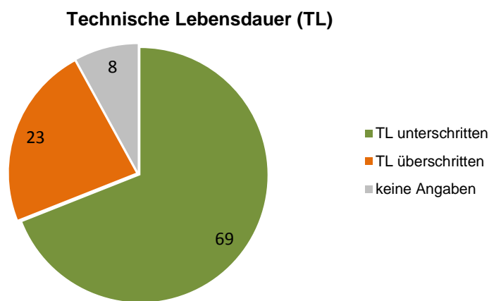
Abb. 82: Über-/Unterschreitung der technischen Lebensdauer (Hauptkomponenten gemäss SIA 382/1) der inspizierten und ausgewählten RLT-Anlagen
