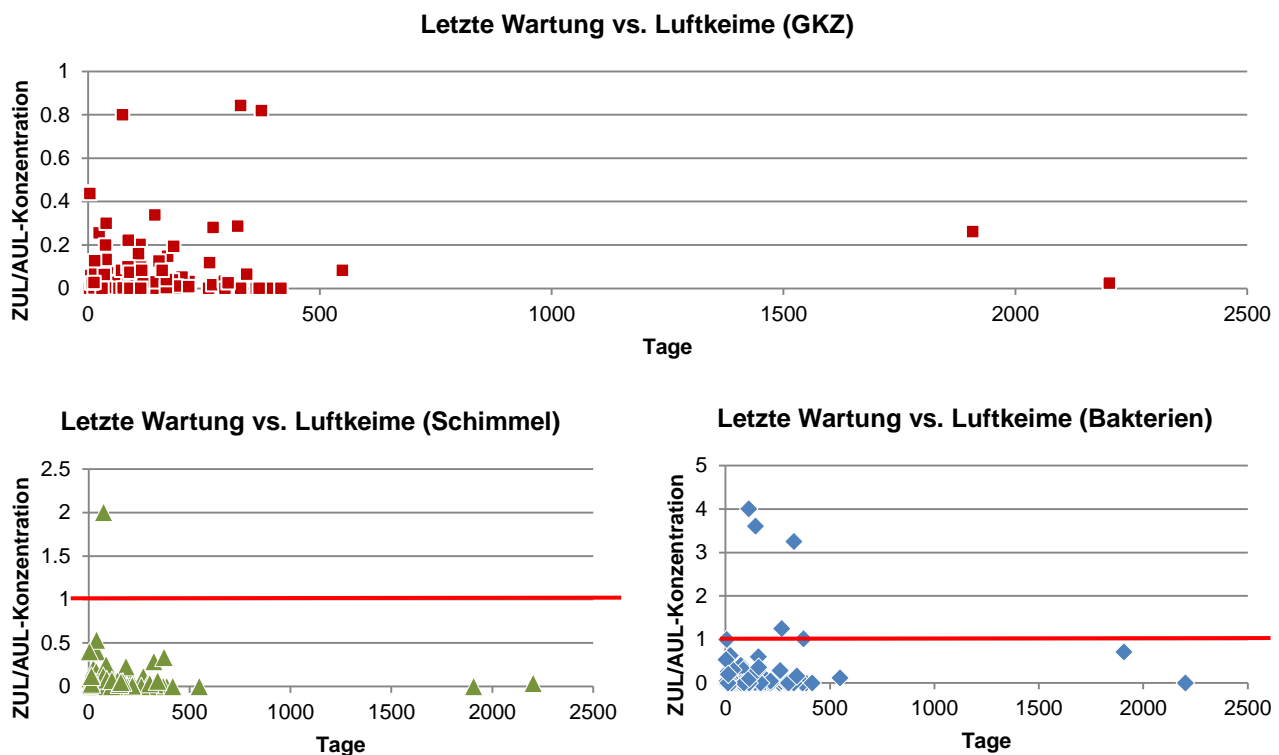
Abb. 72: Verhältnis Zuluft-/Aussenluftkonzentration bezüglich Gesamtkeimzahl (GKZ), Schimmelpilzsporen und Bakterien in Abhängigkeit der letzten Wartung mit Anforderung SWKI-Richtlinie VA104-01 (rote Linie)
