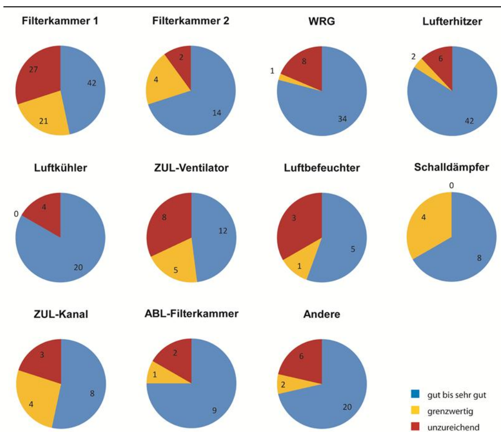
Abb. 11: Beurteilung der Oberflächenkeimuntersuchungen (Beurteilungsschema siehe Anhang) (Andere: weitere Oberflächenkeimuntersuchungen in Zuluftfilter 3, Nachkühler, an Tropfenabscheider etc.)
