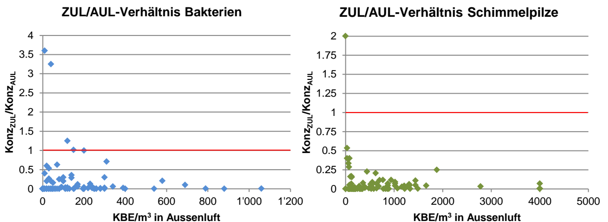
Abb. 19: Verhältnis Zuluft- zu Aussenluftkonzentration bezüglich Bakterien und Schimmelpilzen in Abhängigkeit von der jeweiligen Aussenluftkonzentration dargestellt mit Anforderung (rote Linie) gemäss SWKI VA104-01 (Zuluft gleich/besser Aussenluft)
