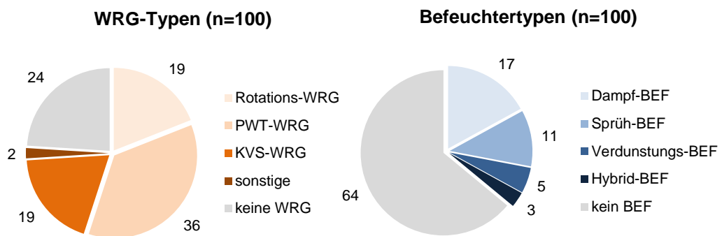
Abb. 8: WRG- und Befeuchter-Typen der inspizierten und ausgewählten RLT-Anlagen
