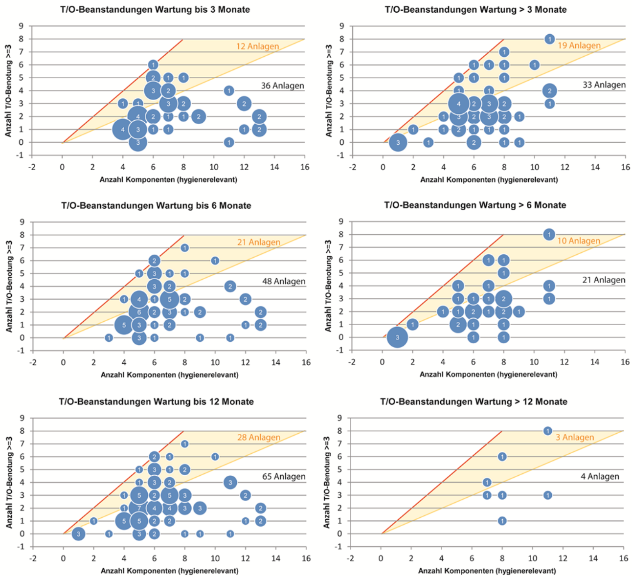
Abb. 70: Anzahl technisch-optische Beanstandungen (ohne unzugängliche Komponenten) in Abhängigkeit zur Gesamtzahl der hygienerlevanten Komponenten der entsprechenden RLT-Anlage und der letzten Wartung.
