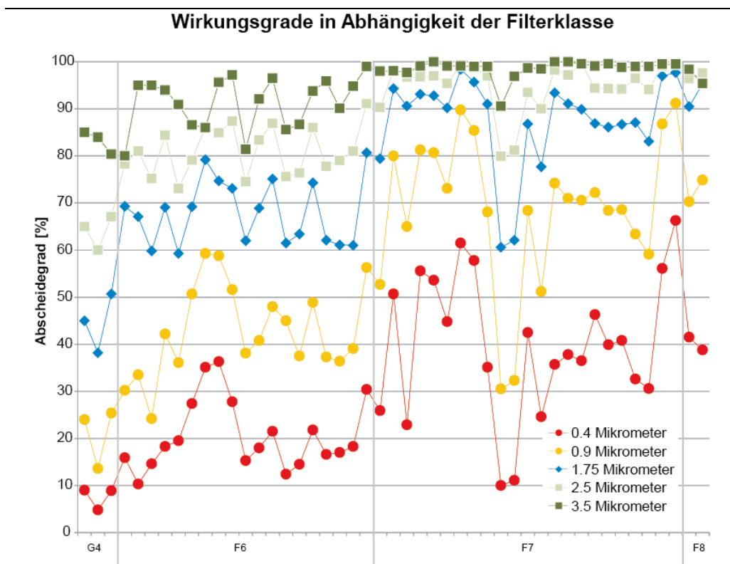
Abb. 54: Gemessene Wirkungsgrade von gebrauchten Filtern
