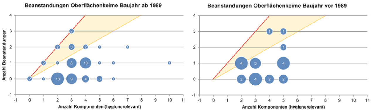
Abb. 68: Anzahl Beanstandungen bezüglich Oberflächenkeimen (Abklatsche und Tupferproben) in Abhängigkeit zur Gesamtzahl der Messorte der entsprechenden RLT-Anlage und zum Anlagenalter. Die Blasenfläche entspricht der Anzahl Anlagen mit gleicher Paarung. Orange hinterlegt: Anlagen, deren Oberflächen zu 50 % und mehr beanstandet wurden. Roter Punkt: Anlagen, die aufgrund fehlender Zugänglichkeit nicht beprobt werden konnten.
