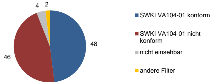
Abb. 87: Erfüllte/Nicht erfüllte Anforderung gemäss SWKI VA104-01 an die letzte Filterstufe (mindestens F7 bzw. F5 bei reinen Umluftanlagen) unter Berücksichtigung aller Baujahre.
