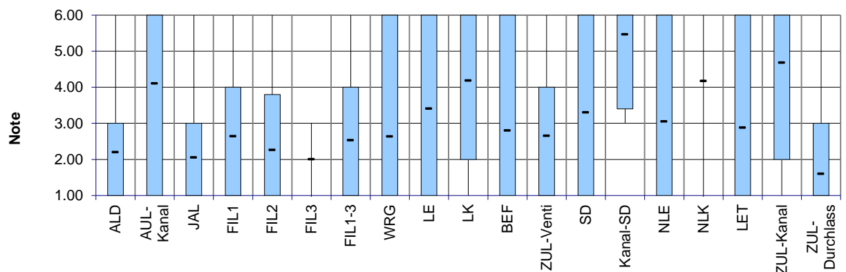
Abb. 26: Statistische Auswertung der T/O-Komponentenbenotung (oben ohne unzugängliche, unten mit unzugänglichen Komponenten).
