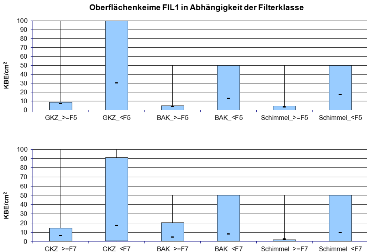
Abb. 49: Statistische Auswertung der Oberflächenkeime (GKZ, Bakterien und Schimmelpilze) in Abhängigkeit der Filterklasse.
