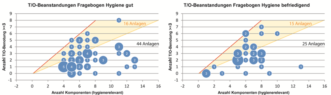
Abb. 73: Anzahl technisch-optische Beanstandungen (ohne unzugängliche Komponenten) in Abhängigkeit zur Gesamtzahl der hygienerelevanten Komponenten der entsprechenden RLT-Anlage und der persönlichen Beurteilung des Hygienezustands durch den Anlagenbetreiber.
