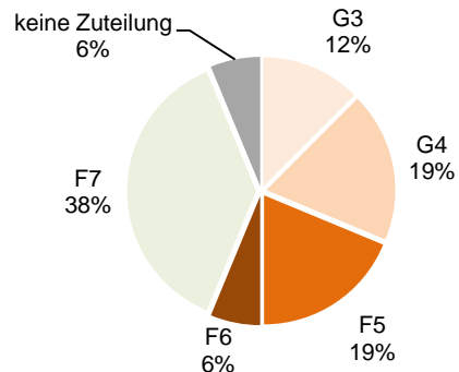
Abb. 43: Klassenverteilung der letzten Filterstufe bei Nichtwohn- und Wohngebäuden
