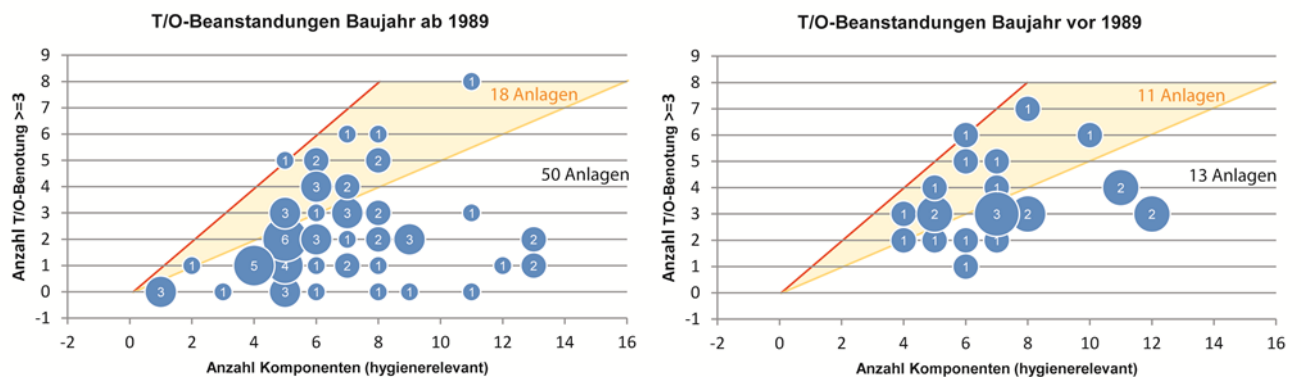
Abb. 63: Anzahl technisch-optische Beanstandungen (ohne unzugängliche Komponenten) in Abhängigkeit zur Gesamtzahl der hygienerelevanten Komponenten der entsprechenden RLT-Anlage und des Anlagenalters.
