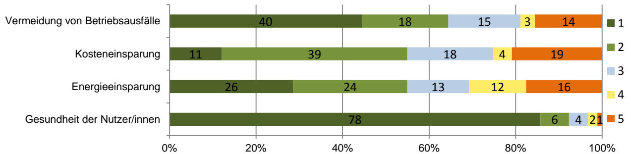
Abb. 16: Beurteilung des Stellenwerts der Anlagenhygiene bezüglich der Vermeidung von Betriebsausfällen, der Möglichkeit zur Kosteneinsparung, der Möglichkeit der Energieeinsparung und der Gesundheit der Nutzer/innen (1=hoch; 5=niedrig).
