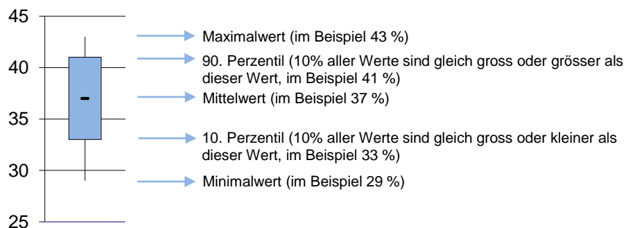
Abb. 25: Interpretationshilfe für statistische Auswertungen (Boxplots)
