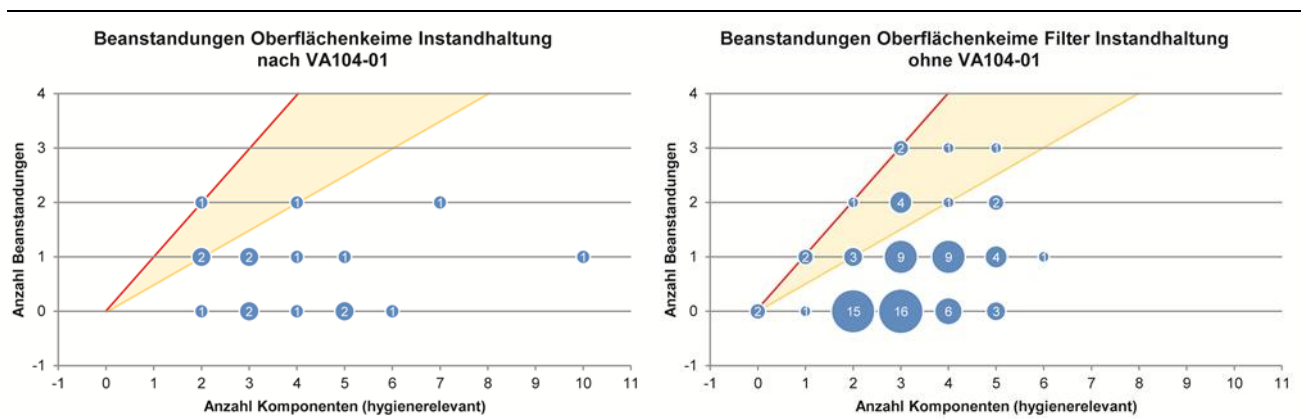
Abb. 81: Anzahl Beanstandungen bezüglich Oberflächenkeimen (Abklatsche und Tupferproben) in Abhängigkeit zur Gesamtzahl der Messorte der entsprechenden RLT-Anlage und der Anwendung der SWKI-Richtlinie VA104-01 bei der Instandhaltung.
