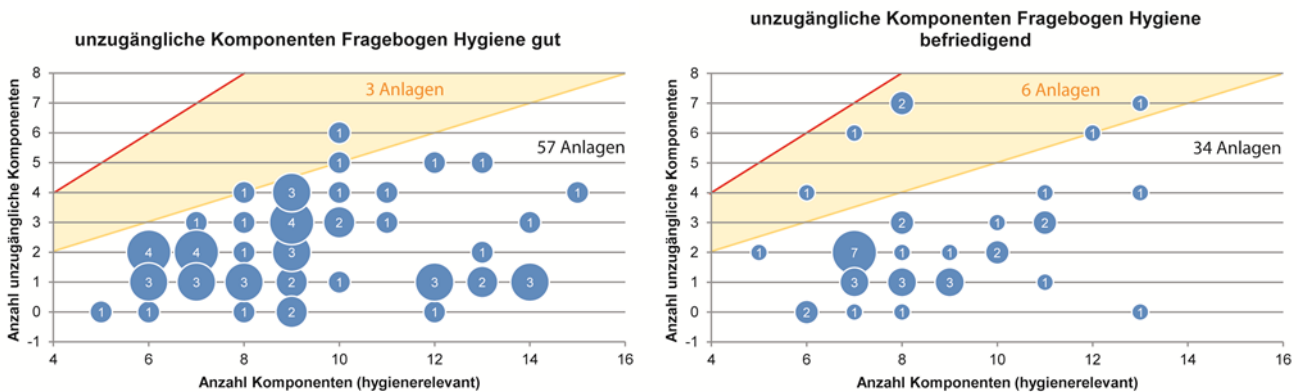
Abb. 76: Anzahl unzugängliche Komponenten in Abhängigkeit zur Gesamtzahl der hygierelevanten Komponenten der entsprechenden RLT-Anlage und der persönlichen Beurteilung des Hygienezustands durch den Anlagenbetreiber.
