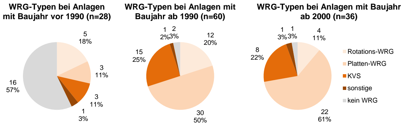
Abb. 83: Verteilung der WRG-Typen in Abhängigkeit vom Baujahr der Anlage
