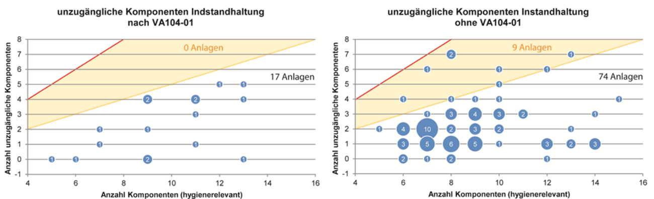
Abb. 78: Anzahl unzugängliche Komponenten in Abhängigkeit zur Gesamtzahl der hygienerelevanten Komponenten der entsprechenden RLT-Anlage und der Anwendung der SWKI-Richtlinie VA104-01 bei der Instandhaltung.
