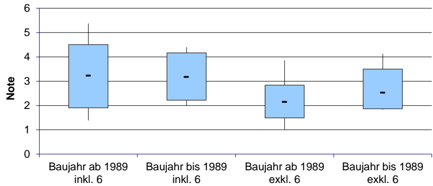
Abb. 62: Statistische Auswertung der T/O-Gesamtnote hygienerelevanter Komponenten in Abhängigkeit vom Anlagenalter (bis 1989/ab1989).
