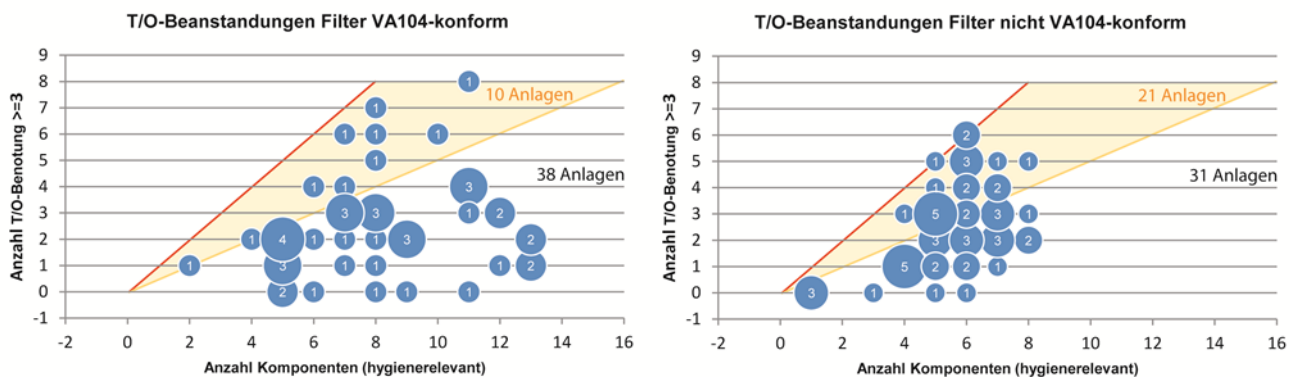
Abb. 46: Anzahl technisch-optische Beanstandungen (ohne unzugängliche Komponenten) in Abhängigkeit zur Gesamtzahl der hygienerlevanten Komponenten der entsprechenden RLT-Anlage und der Frage, ob die Filterklasse Richtlinienkonform ist.
