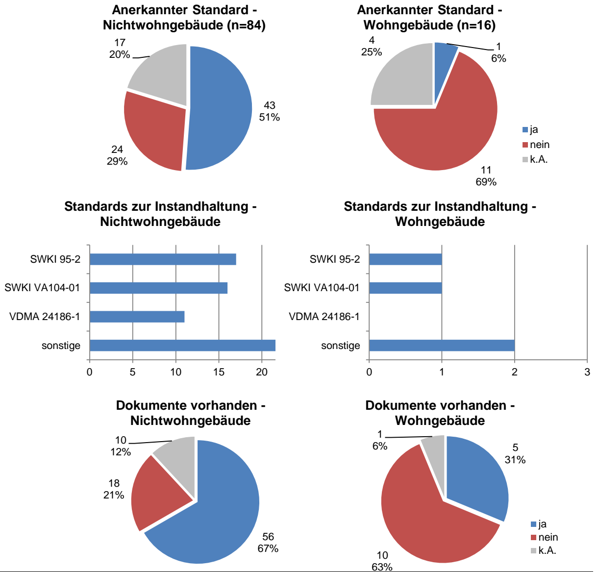
Abb. 45: Angaben zur Instandhaltung durch Anlagenverantwortliche von Wohn- und Nichtwohngebäuden
