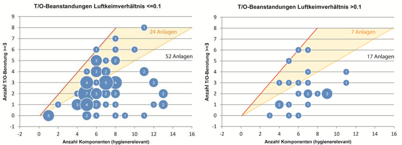
Abb. 59: Anzahl technisch-optische Beanstandungen (ohne unzugängliche Komponenten) in Abhängigkeit zur Gesamtzahl der hygienerlevanten Komponenten der entsprechenden RLT-Anlage und des Luftkeimverhältnisses.
