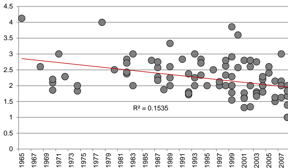
Abb. 64: Technisch-optische Beurteilung aller untersuchter RLT-Anlagen in Abhängigkeit des Baujahrs
