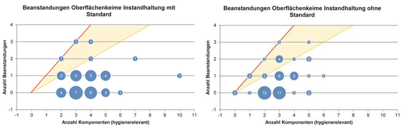
Abb. 80: Anzahl Beanstandungen bezüglich Oberflächenkeimen (Abklatsche und Tupferproben) in Abhängigkeit zur Gesamtzahl der Messorte der entsprechenden RLT-Anlage und der Anwendung eines anerkannten Standards bei der Instandhaltung. Die Blasenfläche entspricht der Anzahl Anlagen mit gleicher Paarung. Orange hinterlegt: Anlagen, deren Oberflächen zu 50 % und mehr beanstandet wurden. Roter Punkt: Anlagen, die aufgrund fehlender Zugänglichkeit nicht beprobt werden konnten.
