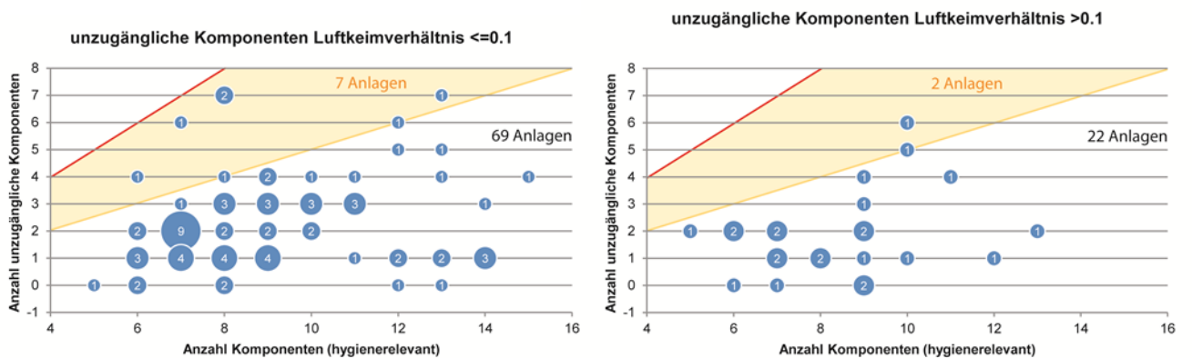
Abb. 60: Anzahl unzugängliche Komponenten in Abhängigkeit zur Gesamtzahl der hygienerlevanten Komponenten der entsprechenden RLT-Anlage und des Luftkeimverhältnisses.
