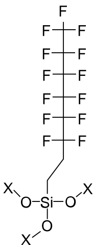
Abb. 1: Strukturformel eines Fluoralkylsilanols ( X = \text{Alkylgruppe} oder \text{Wasserstoff} ) mit der Summenformel: \text{C}_6\text{F}_{13}(\text{C}_2\text{H}_4)_n\text{Si}(\text{OH})_n(\text{O-Alkylgruppe})_{3-n} (mit 0 \leq n \leq 3 ).
